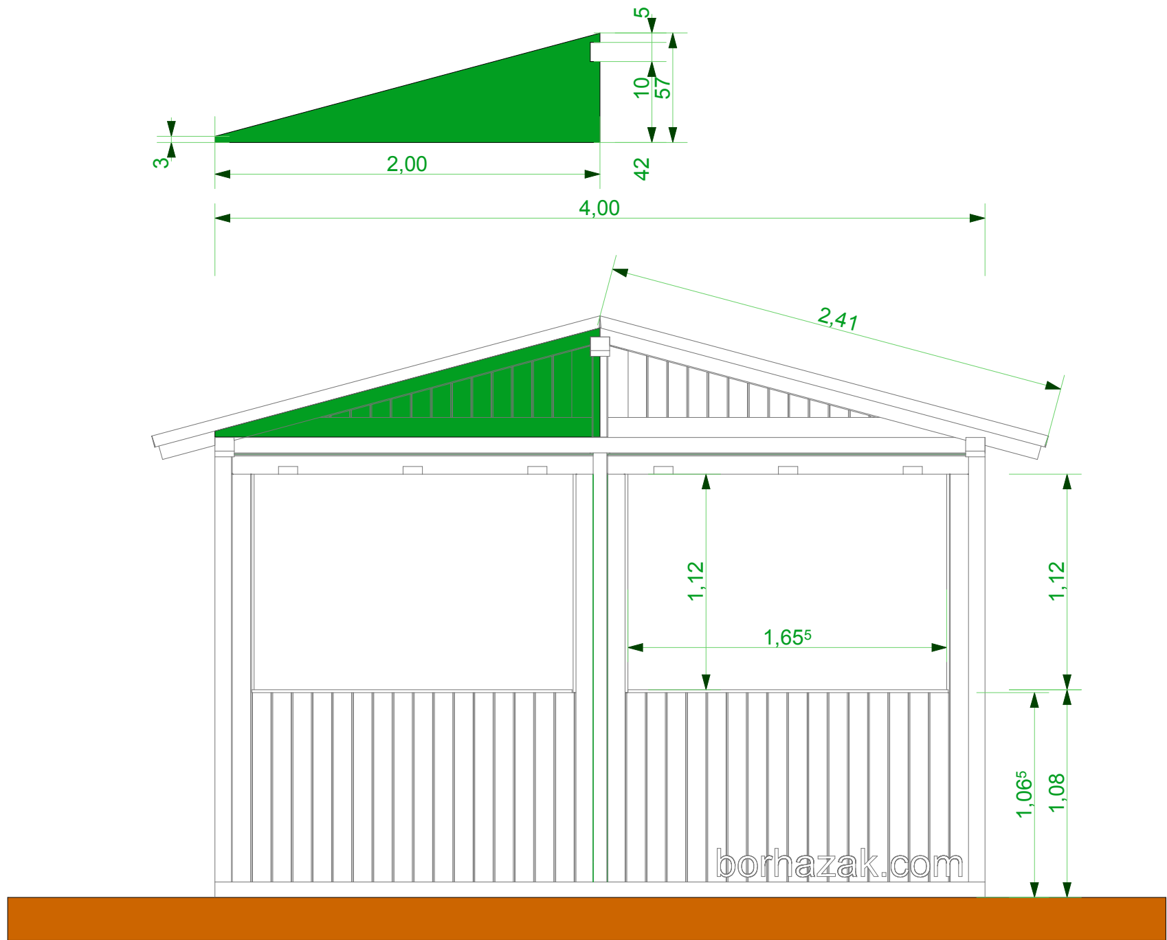
4x2 és 4x4 méteres faház homlokzata
